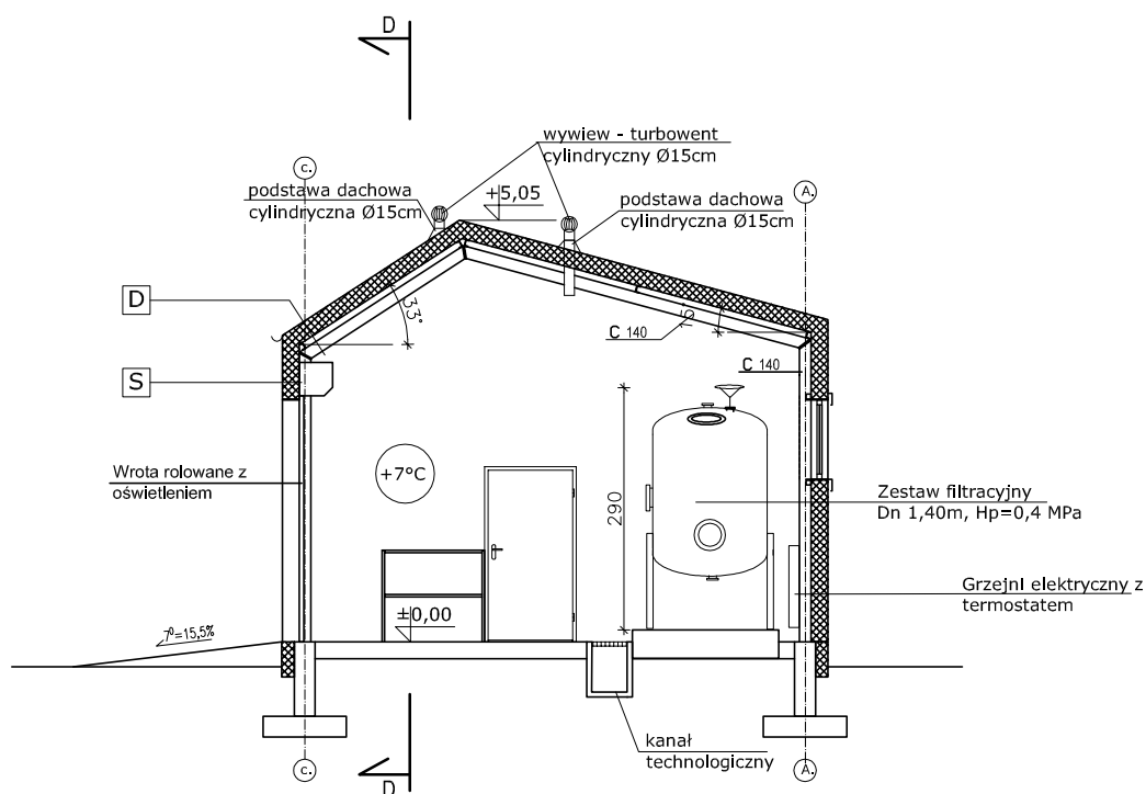
Przekrój C-C
