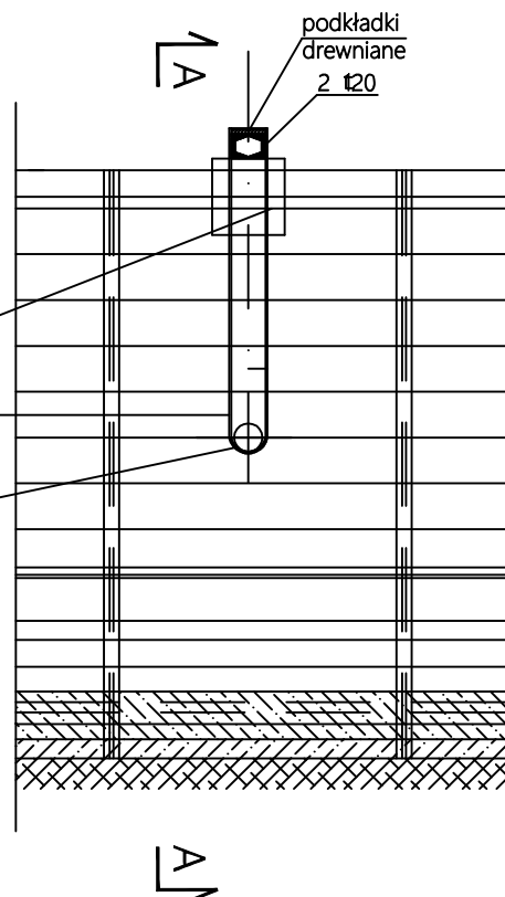
Przekrój B-B
