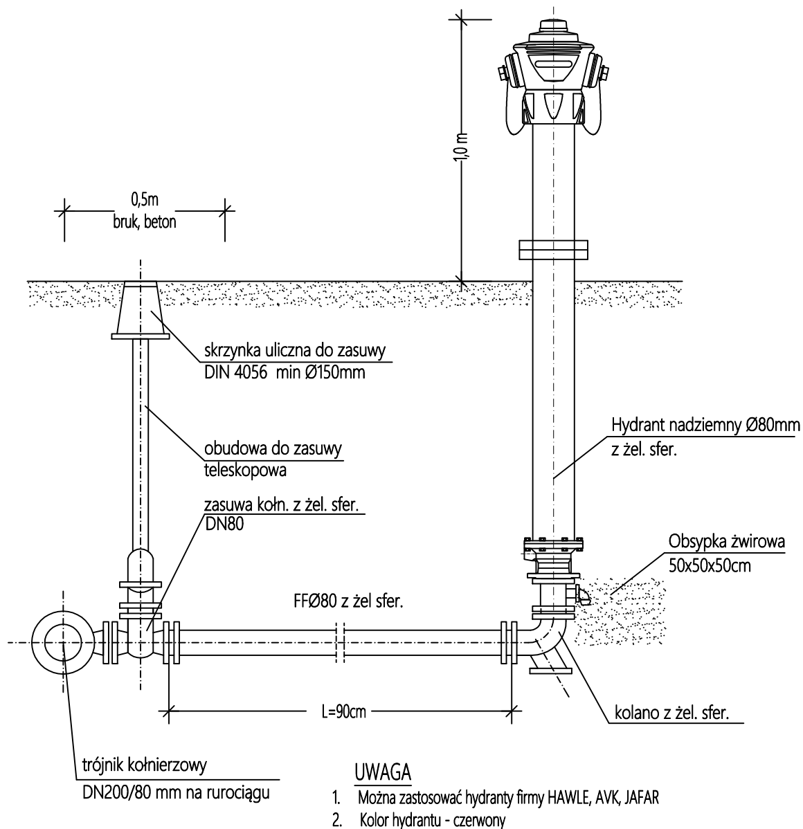
Schemat montażowy
