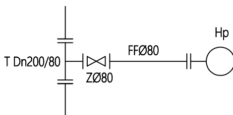
Schemat montażowy
